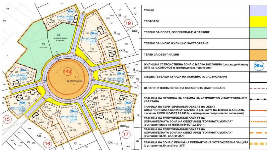
Фиг. 15. ПУП – ИПРЗ за „Голямата могила“, с. Продановци – чертеж „ПЗ“
