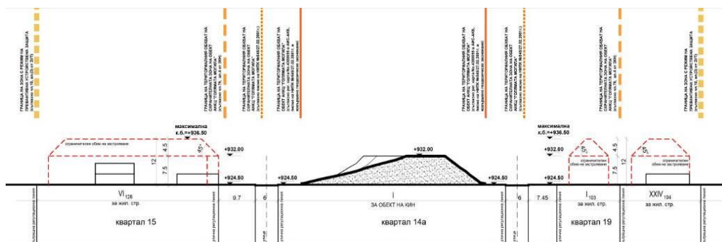
Фиг. 16. ПУП – ИПРЗ за „Голямата могила“, с. Продановци – чертеж „РУП – силует/разрез“
